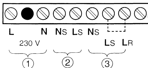
Joonis 13. Toitepinge ühenduse klemmiplaat
