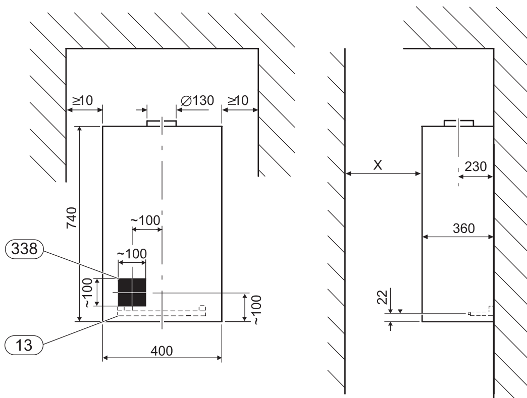
Joonis 1. Vaade eest ja küljelt
