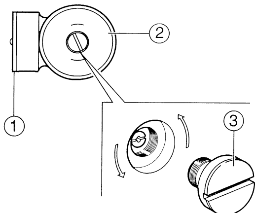
Joonis 21. Õhu eemaldamine/pumba lahtiblokeerimine
