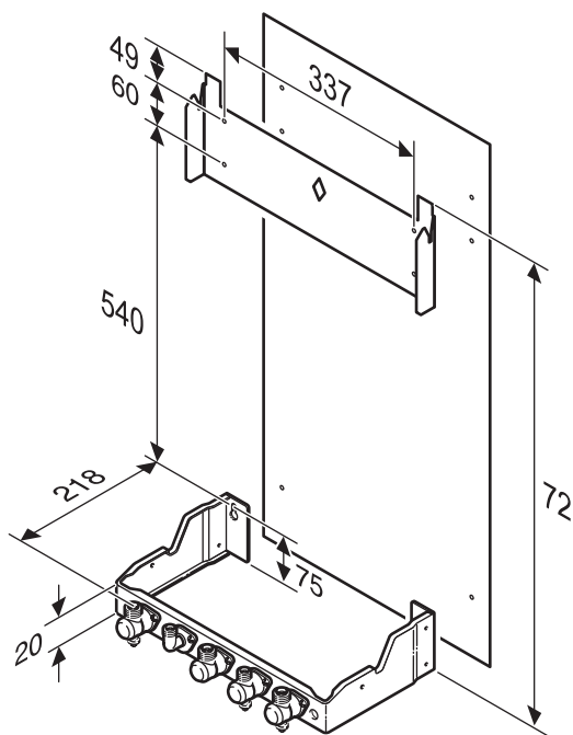
Joonis 5. Paigaldamine seinale
