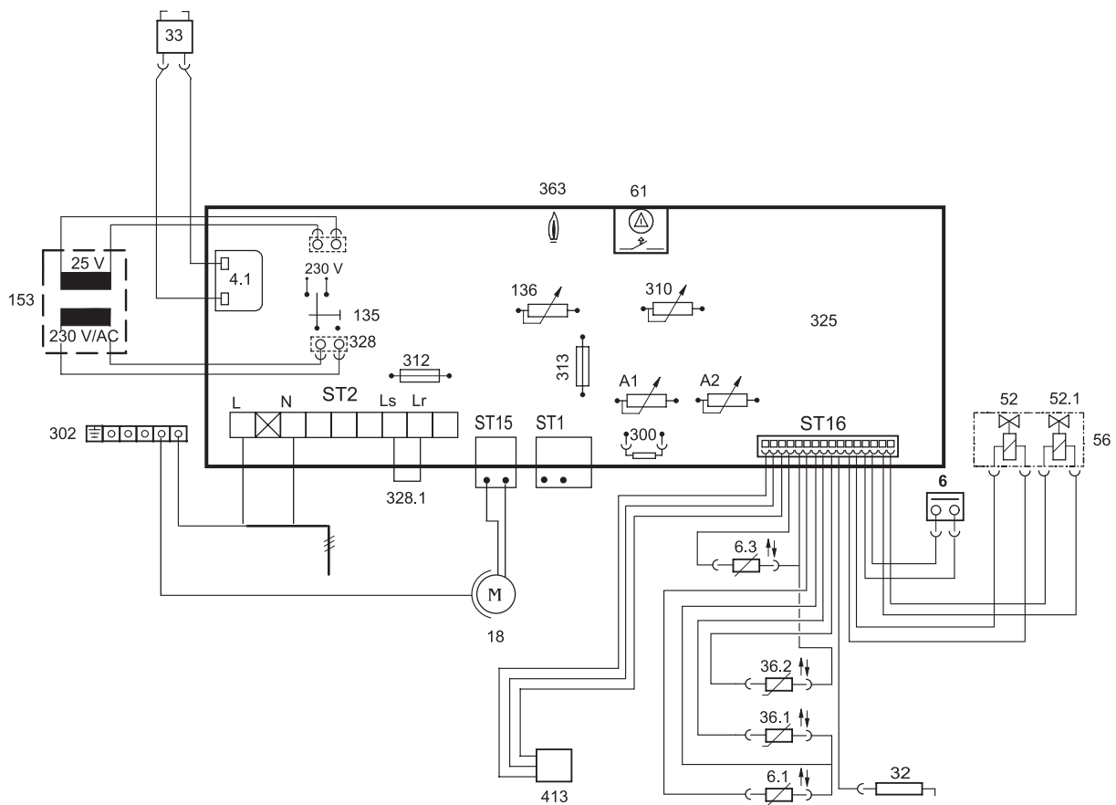
Joonis 2. Elektriskeem
