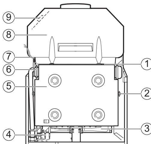
Joonis 40. Kaitse-ekraani taga olevad osad
