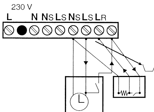
Joonis 17. Ruumitemperatuuri regulaatori 230 V ja taimeri 230 V ühendamine (eemaldada sild L_S ja L_R vahel)
