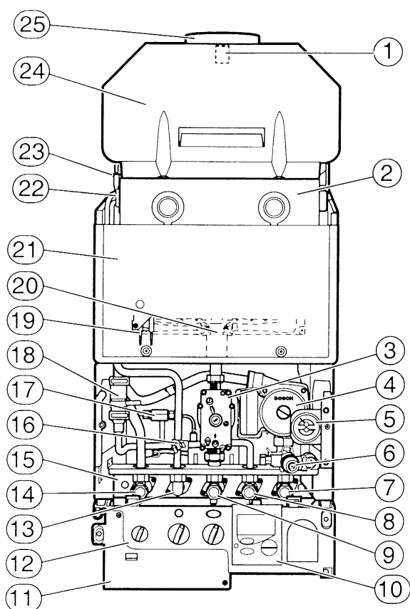
Joonis 19. Seadme ehitus, Eurotronic on hooldusasendis
