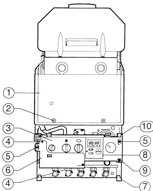
Joonis 38. Põlemiskambri kaitse-ekraani ja Eurotronic kinnitus
