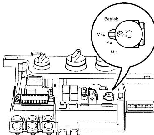
Joonis 26. Töörežiimi seadmine
