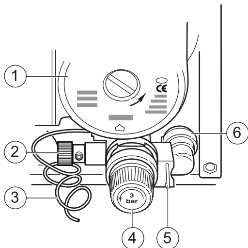
Joonis 22. Kaitseventiil
