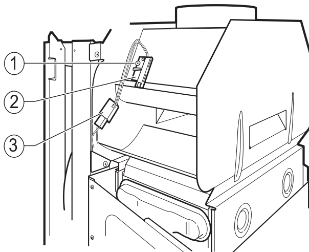
Joonis 41. Tõmbekontrolli sond
