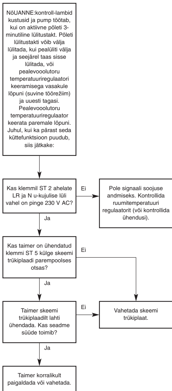
Joonis 46, test B
