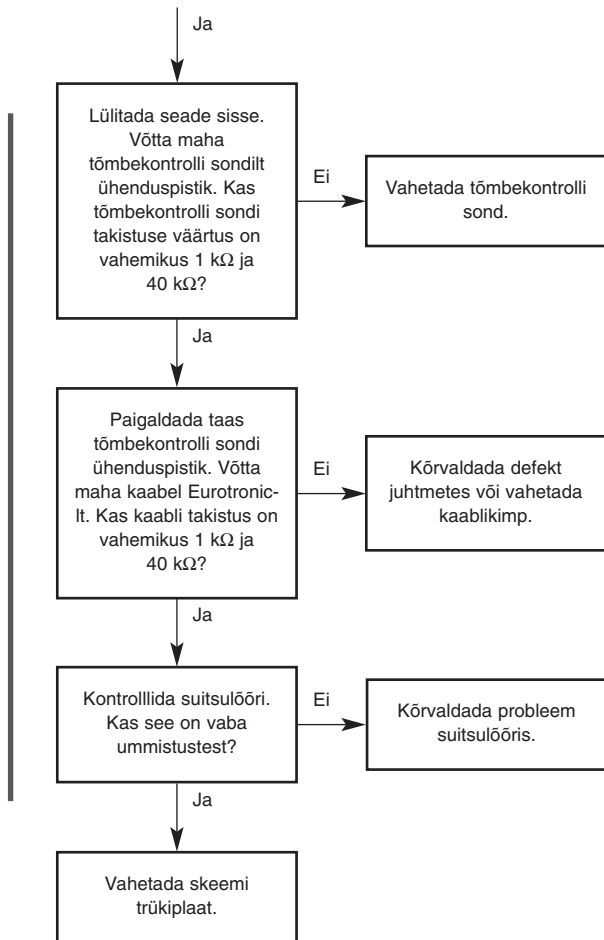
Joonis 51, test E (osa 2)
