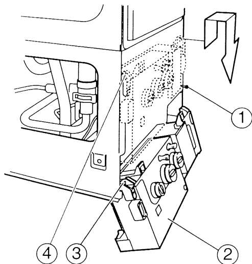
Joonis 39. Eurotronic paigutamine hooldusasendisse
