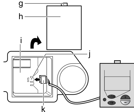
Joonis 18. Kaas
