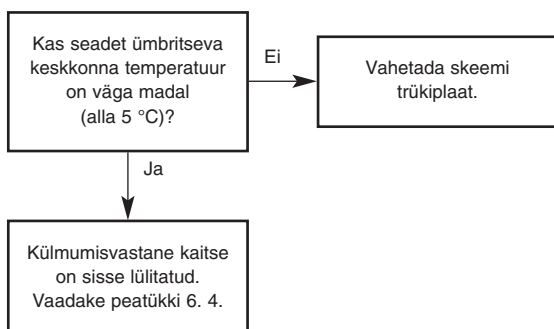
Joonis 53, test G
