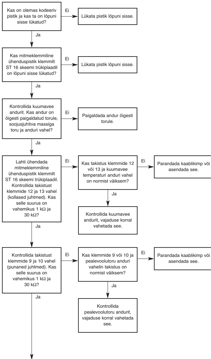
Joonis 50, test E (osa 1)
