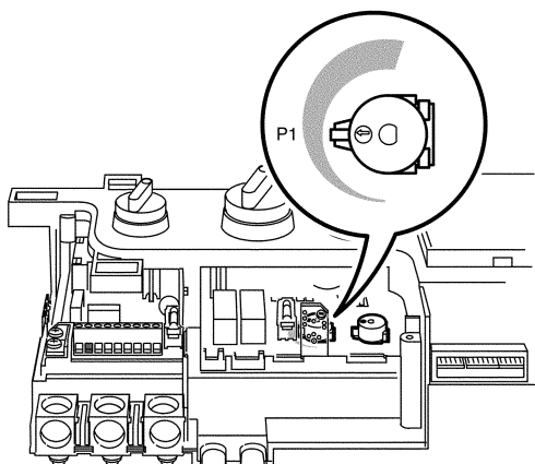
Joonis 27. Maksimaalse soojusvõimsuse seadmine
