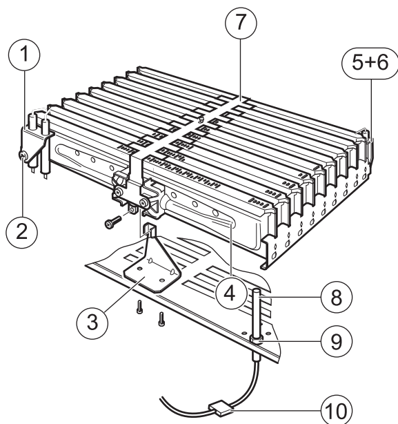
Joonis 42. Põletite plokk
