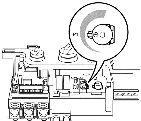
Joonis 23. Pumba lülitusmooduse seadmine
