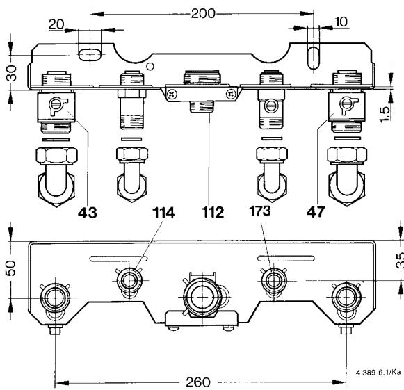
Joonis 7. Torustike külge ühendamine
