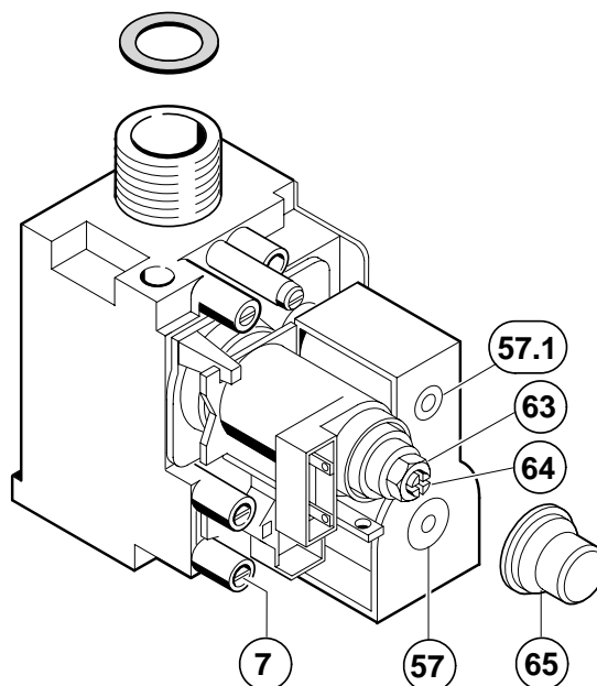
Joonis 42. Gaasiarmatuur
