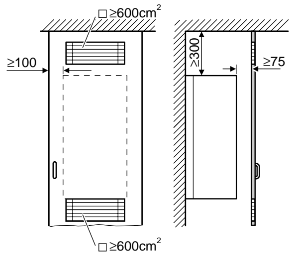
Joonis 5. Õhu juurdepääsuavad seadme paigaldamisel kappi
